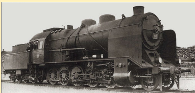
Die LBE-Lokomotive 100, eine schwere Lok von 1936.
