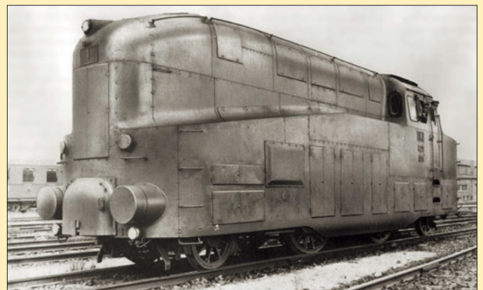
Stromlinienverkleidete Lokomotive Nr. 1 der LBE 1936.
